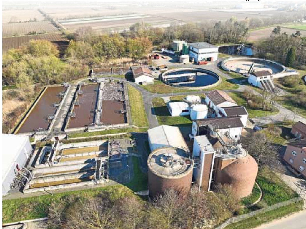
Mitte September 1972 wurde Richtfest für den Neubau der Kläranlage gefeiert. Seither wurde das Klärwerk erweitert, erneuert und modernisiert, ist im Kern aber noch die Anlage von 1972.
